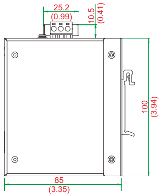
左侧视图
